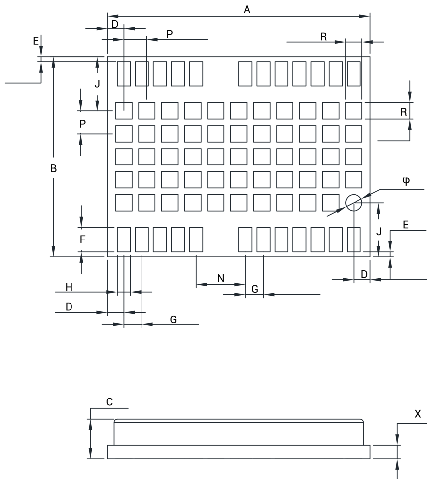
图 2-2 UM960E机械图
