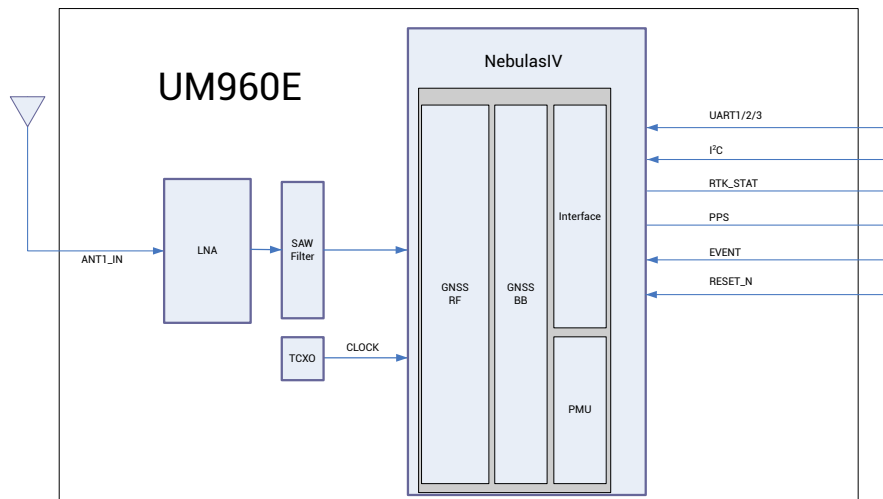
图 1-2 UM960E结构框图
