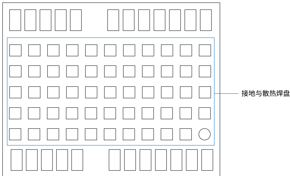
图 3-3 UM960E接地与散热焊盘（底视图）
