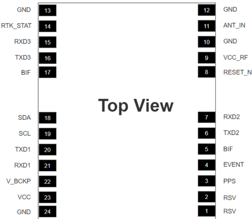
图 2-1 UM960E引脚图
